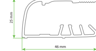
DESIGN PURE YP Dönüş Profili
