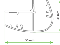
DESIGN AK - DESIGN SAK - AURA SAK YP Dönüş Profili
