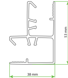
AURA KY SOLVA YP Dönüş Profili
