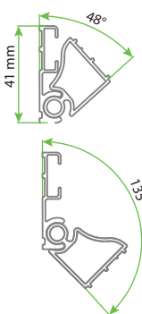
Mafsallı Profil Seti
