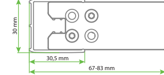
DESIGN PURE AK Duvar Dikme Ayar Profili
