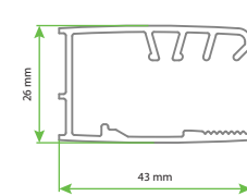
8mm Duvar Dikme Profili
