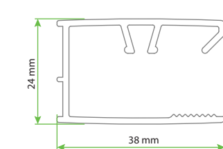
SOLVA / AURA PURE SAK Duvar Dikme Profili
