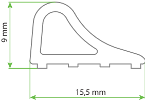
XTENSA AQUANIT Tekne İçin Yan Panel Alt Ray Profili
