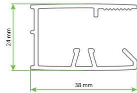
DESIGN PURE SAK Duvar Dikme Profili
