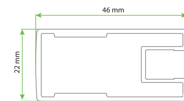
AURA KY SOLVA YP Dönüş Profili
