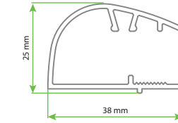
DESIGN AK YP Dönüş Profili
