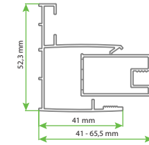
X1 - X0 - CLASSICS PS X1 EASY ENTRY Kulaklı Duvar Dikme Ayar Profili
