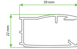
CLASSICS KY C YPT Duvar Dikme
