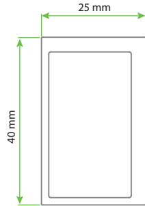
40X25 CM Kutu Profili
