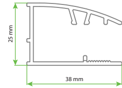
DESIGN - AURA SAK Duvar Dikme
